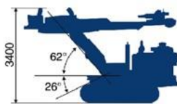
3. Угол наклона буровой штанги
