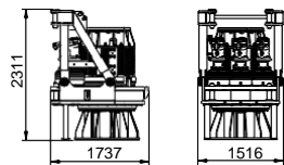
Вращательно-буравная головка
